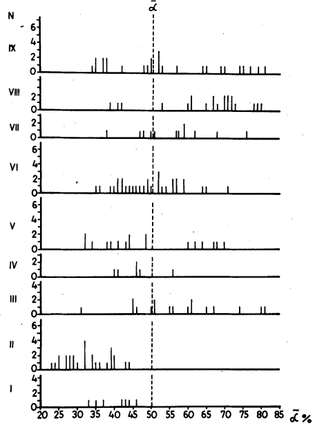
(d) Groundwater recharge coefficient.
