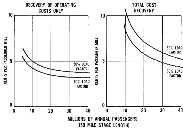
Fig. 17 TLV breakeven fare
