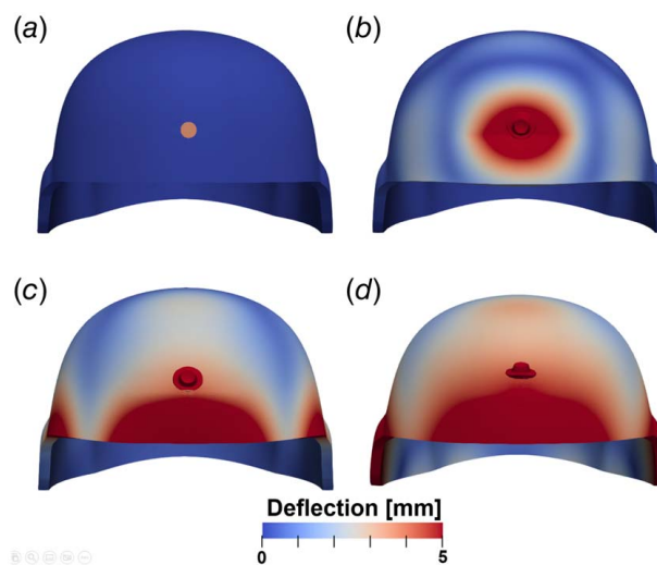
Fig. 5 Helmet shell deflection at (a) 0 \mu s, (b) 12 \mu s, (c) 25 \mu s, and (d) 50 \mu s
