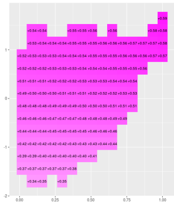
(a) BLEU
