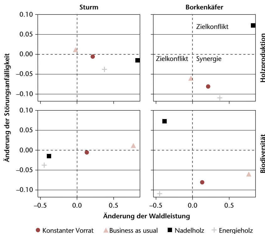
Abb 5 Zielkonflikte und Synergien zwischen Waldleistungen (Holzproduktion, Biodiversität) und Störungsanfälligkeit (Sturm, Borkenkäferbefall). Die Achsenwerte zeigen die proportionalen Veränderungen gegenüber dem Jahr 2016, die über die Jahre 2026–2106 gemittelt wurden.
