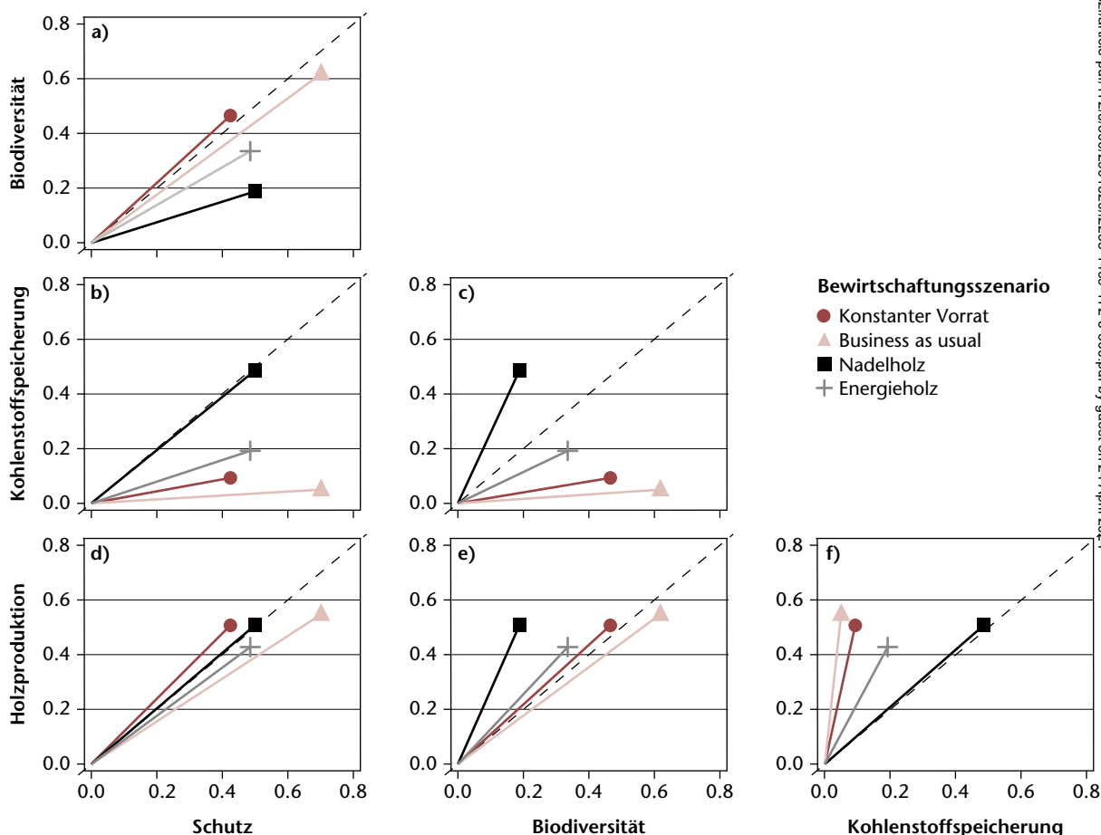
Abb 3 Paarweise Darstellung von Waldleistungen, um Zielkonflikte zu ermitteln. Die Position der Symbole repräsentiert über die Simulationsperiode gemittelte Teilnutzen. Je grösser der Abstand von der 1:1-Linie (gestrichelt) ist, desto grösser ist der Zielkonflikt zwischen den zwei Waldleistungen. Der Abstand vom Ursprung (durchgezogene Linie) steht für den kombinierten Nutzen der beiden Waldleistungen.
