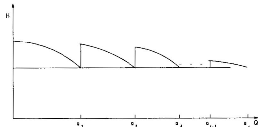
Figura 1. Bombas en paralelo
