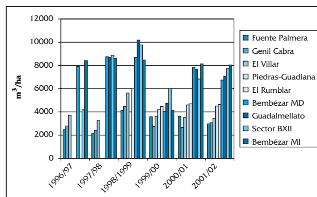
Figura 3. Suministro de agua de riego por unidad de área regada (m 3 /ha)
