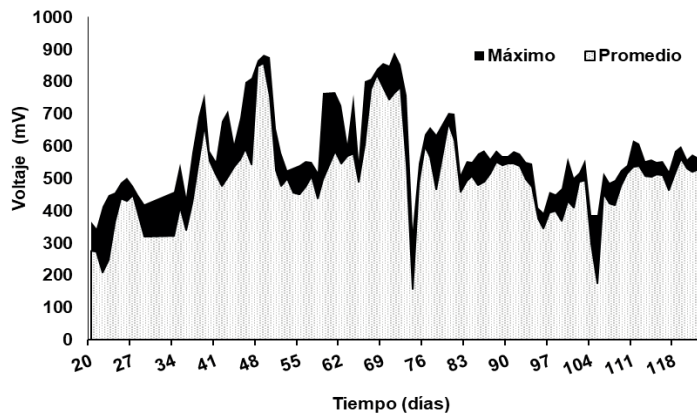
Figura 5 | Voltajes máximo y promedio diarios generados por HC-CCM con flujo continuo ascendente.
