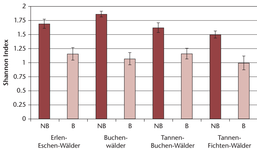
Abb 6 Shannon-Index für die Habitatstrukturen, nach Waldtyp und nach Bewirtschaftungsmodus aufgeteilt. Mittelwerte mit Standardfehlern. Alle Unterschiede «bewirtschaftet» – «nicht bewirtschaftet» sind statistisch signifikant (Mann-Whitney-U-Test: p < 0.05 ).
