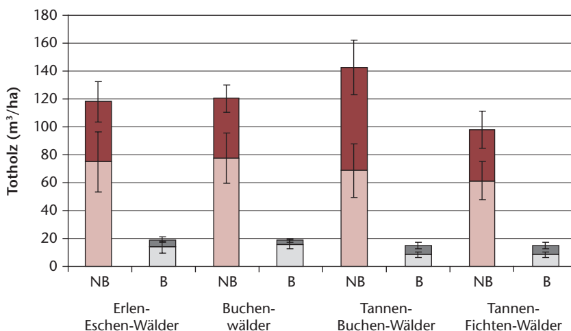
Abb 4 Volumen von stehendem und liegendem Totholz in den vier verschiedenen Waldtypen. NB: Wälder ohne Bewirtschaftung, B: Wälder mit Bewirtschaftung. Rosa und hellgrau: liegendes Totholz, rot und grau: stehendes Totholz. Mittelwerte und Standardfehler. Alle Unterschiede NB–B statistisch hoch signifikant.
