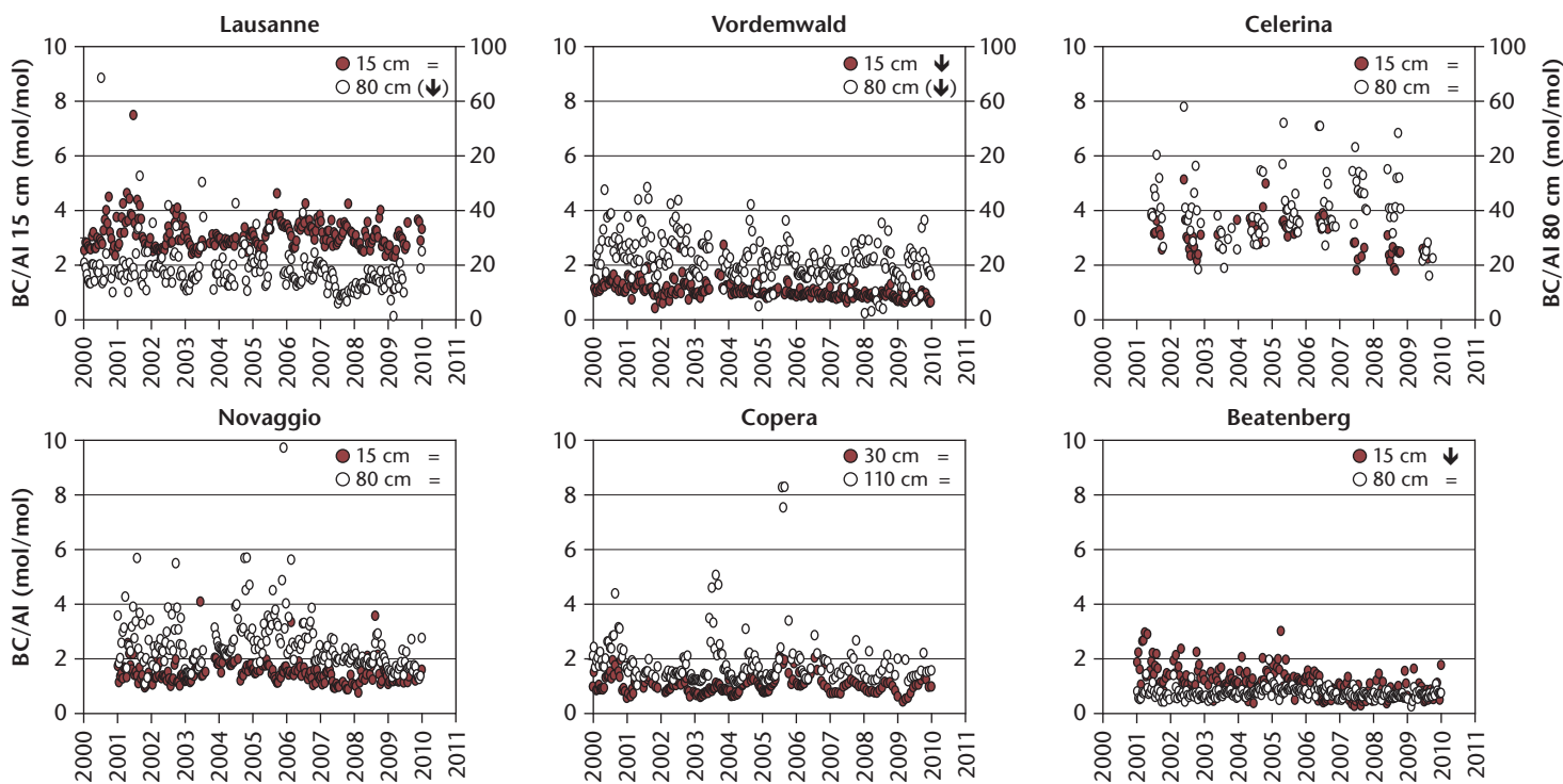
Fig. 6 Séries temporelles des rapports BC/Al (mol/mol) dans les solutions du sol à 15 cm et 80 cm de profondeur depuis 2000 (ou plus tard) jusqu'en 2009. A Lausanne, Vordemwald et Celerina, l'échelle des rapports BC/Al à 80 cm de profondeur se trouve sur l'axe à droite du graphique. Les tendances temporelles (voir tableau 2) sont indiquées dans la légende: = pas de tendance; (v) diminution peu significative (p < 0.05); (v) diminution significative (p < 0.01).
