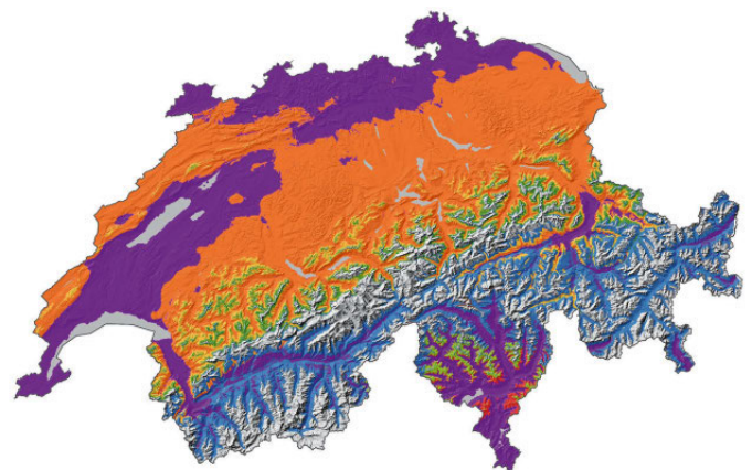
Vegetationshöhenstufenkarte Periode 2070–2099 (CLM-Modell)
