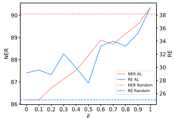
(b) WebNLG
