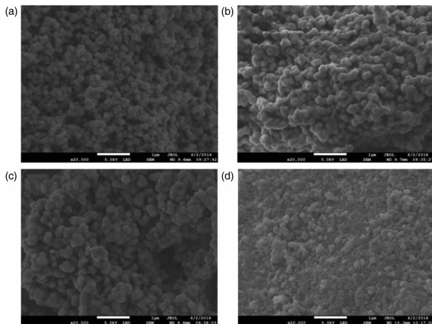
Figure 4 | SEM images of (a) MPs, (b) SCMPs, (c) PSCMPs-NH 2 , (d) PSCMPs-NH 2 -TiO 2 /Ag.
